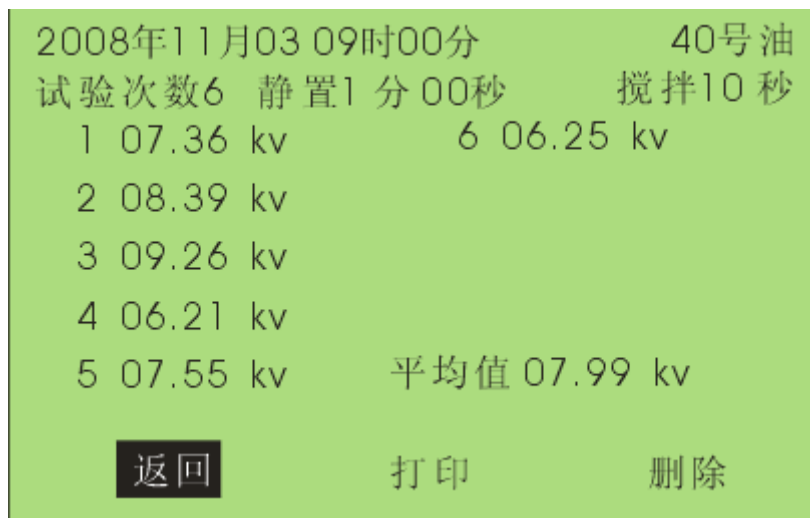
图 2.8 击穿试验结果显示
