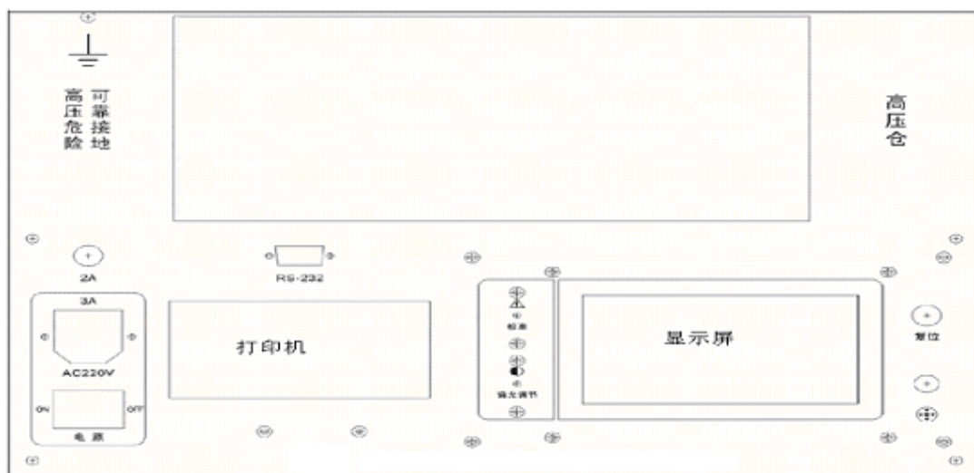
图 1.1 绝缘油耐压测试仪面板
